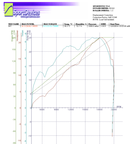
Gambar 5 Grafik data saat menggunakan knalpot standart
