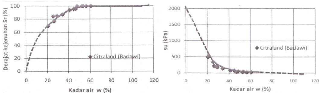
Gambar 1. Variasi Kekuatan Geser, Kadar Air, dan Derajat Kejenuhan.
