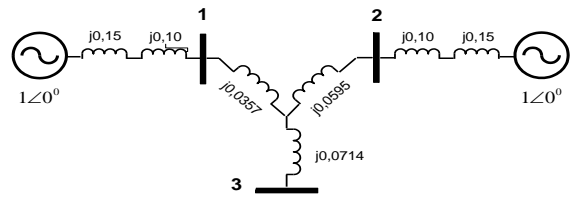
Gambar-3. Diagram ekuivalen impedansi urutan positif
