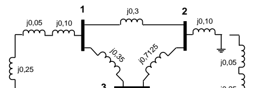
Gambar-6. Diagram impedansi urutan nol Menentukan impedansi Thevenin yang dipandang dari bus gangguan (bus 3), dengan mengubah bentuk segitiga bus 123 menjadi ekuivalen bintang.
