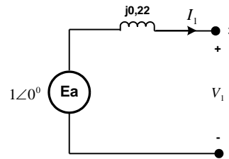
Gambar-4. Jaringan urutan positif Menentukan impedansi urutan negatif setiap elemen yang mana nilainya sama dengan impedansi urutan positifnya.
