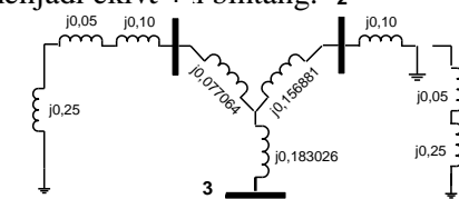
Gambar-7. Diagram ekuivalen impedansi urutan nol
