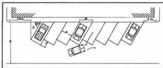
Gambar 3. Pola parkir menyudut 60°
