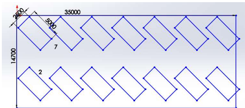
Gambar 9. Kapasitas Mobil pada Mirota Kampus dengan Sudut 45°
