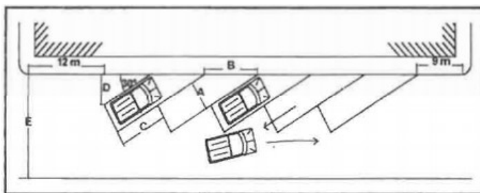
Gambar 1. Pola Parkir Menyudut 30°
