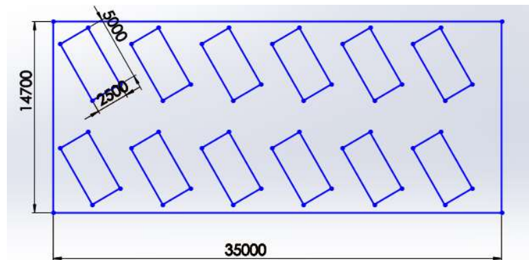
Gambar 13. Kapasitas Mobil pada Mirota Kampus dengan Sudut 30^\circ
