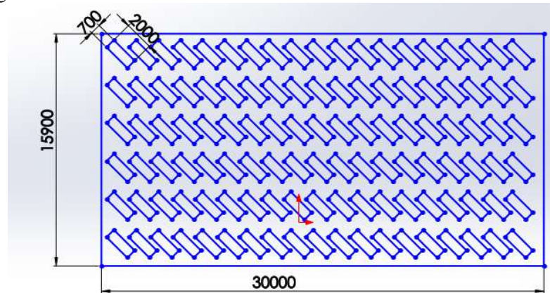
Gambar 8. Kapasitas Motor pada Mirota Kampus dengan Sudut 45°
