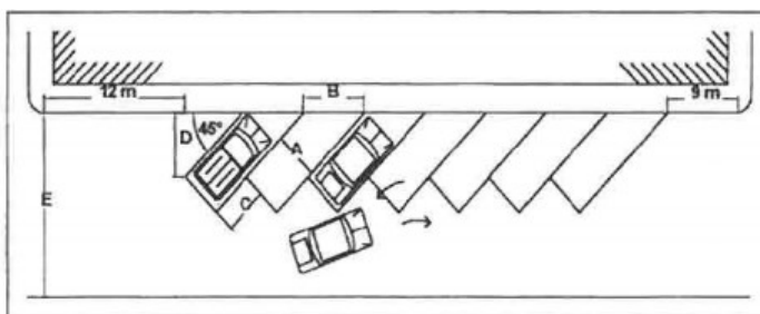
Gambar 2. Pola parkir menyudut 45°
