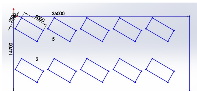
Gambar 11. Kapasitas Mobil pada Mirota Kampus dengan Sudut 60^\circ
