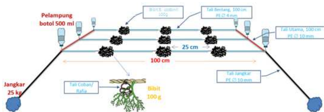
Gambar 1. Konstruksi budidaya rumput laut metode longline .
