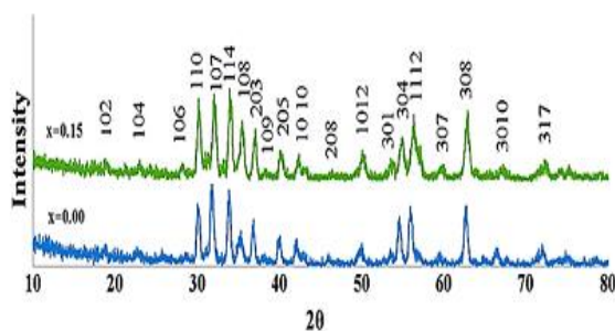
Gambar 11. Pola difraksi XRD \text{Ba}_{(1-2x)}\text{La}_x\text{Na}_x\text{Fe}_{10}\text{CoZrO}_{19} ( x=0,00 , dan 0,15 )
