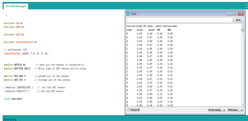
Gambar 6. Hasil pengujian dengan Modul Micro SD Card
