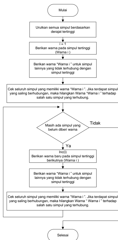
Gambar 6. Algoritma Welch-Powell yang telah Dimodifikasi
