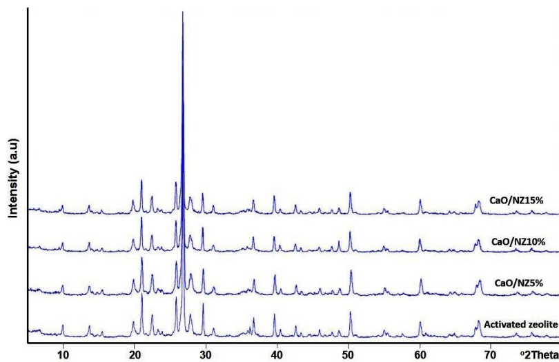
Gambar 4. Pola difraksi sinar-X katalis CaO/zeolit alam
