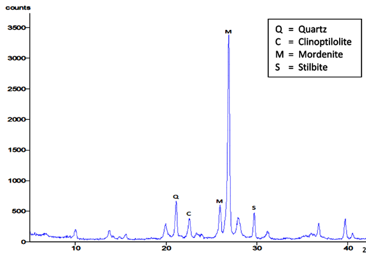
Gambar 2. Pola difraksi sinar-X zeolit alam
