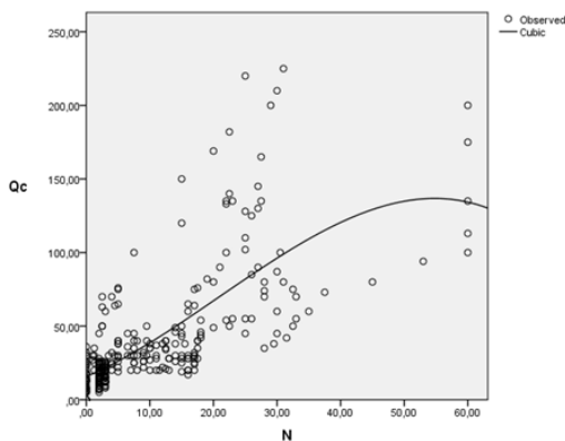
Gambar 5. Garis Regresi Kubik q_c dengan N Menggunakan Program SPSS
