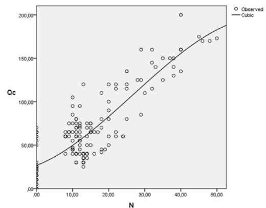
Gambar 6. Garis Regresi Kubik q_c dengan N Menggunakan Program SPSS
