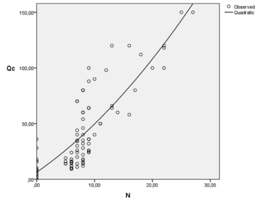
Gambar 4. Garis Regresi Kuadratik q_c dengan N Menggunakan Program SPSS Sumber : Data diolah, 2017
