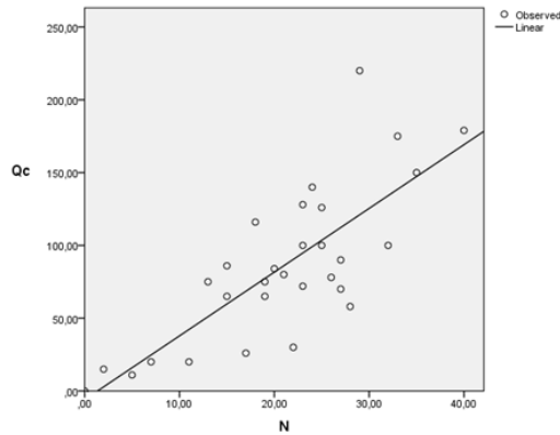
Gambar 3. Garis Regresi Linier q_c dengan N Menggunakan Program SPSS Sumber : Data diolah, 2017
