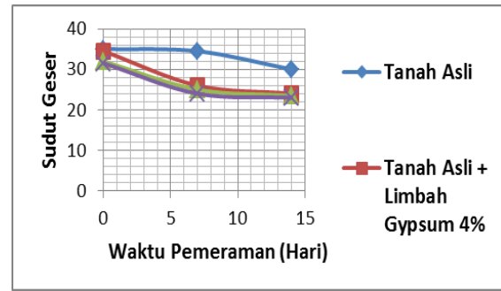
Gambar 7. Grafik nilai sudut geser
