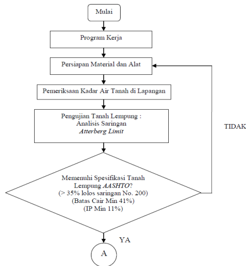
Gambar 1. Diagram alir pengujian klasifikasi tanah
