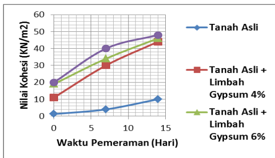
Gambar 6. Grafik nilai kohesi
