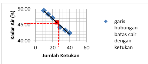
Gambar 4. Grafik hasil pengujian batas cair
