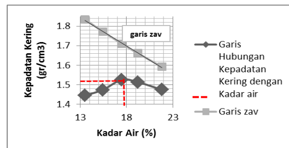
Gambar 5. Grafik hasil pengujian pemadatan
