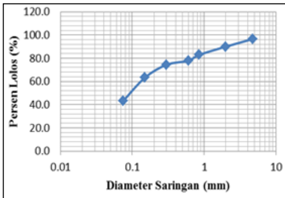
Gambar 3. Grafik hubungan persentase lolos dengan diameter saringan
