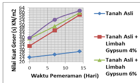
Gambar 8. Grafik nilai kuat geser
