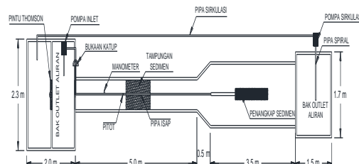
Gambar 2. Denah Flushing Conduit
