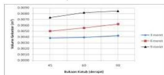
Gambar 9. Grafik pengaruh bukaan katub terhadap volume gelontor pada panjang pipa isap 0,5 cm
