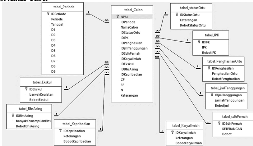
Gambar 3. Relasi Tabel
