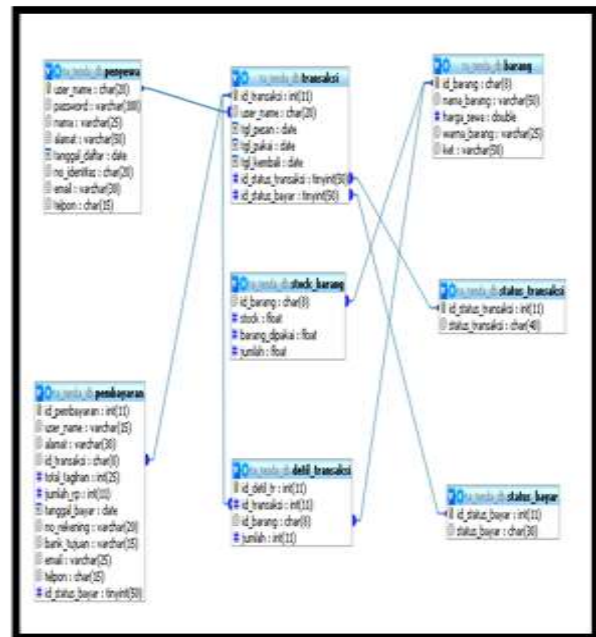
Gambar. Relasi Antar Tabel Sistem Informasi penyewaan dan pemesanan tenda
