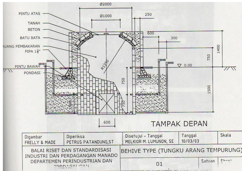
Gambar 3. Tungku pembuatan arang tempurung tipe beehive
