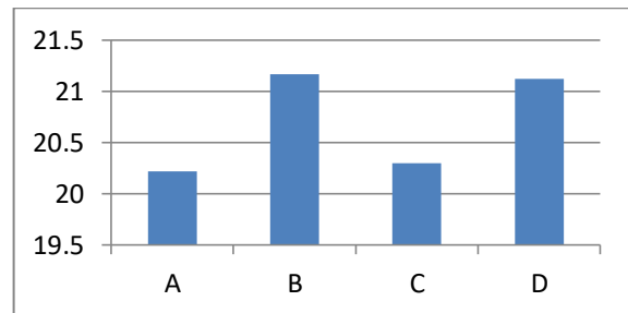
Gambar 3. Pengaruh perlakuan daerah pengambilan contoh terhadap bahan mudah menguap pada suhu 950 °C dari produk arang aktif tempurung kemiri.
