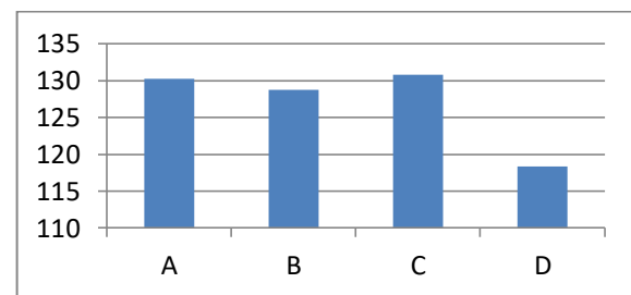
Gambar 6. Pengaruh perlakuan daerah pengambilan contoh terhadap daya serap biru metilena dari produk arang aktif tempurung kemiri
