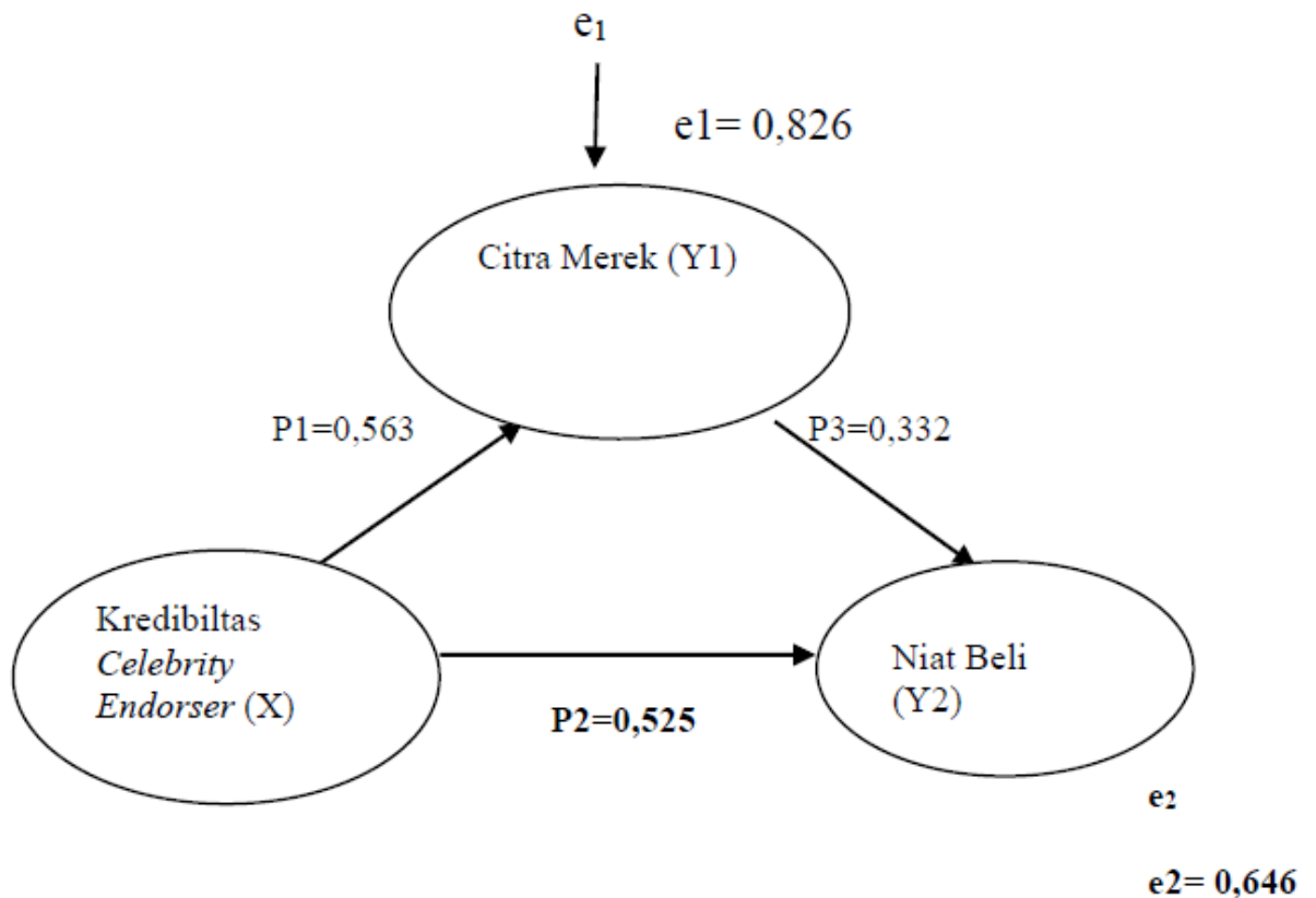
Gambar 2. Validasi Model Diagram Jalur Akhir
