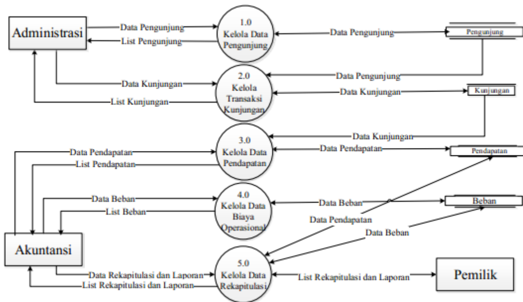
Gambar 1.4 DFD Level- 0 Aplikasi Sistem Perhitungan Laporan Laba Rugi Menggunakan Metode Single Step.
