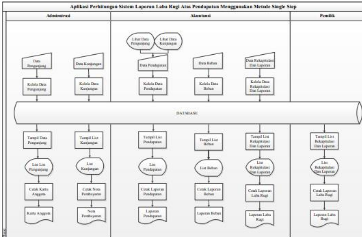
Gambar 1.2 Flowmap Prosedur Perhitungan Sistem Laporan Laba Rugi Menggunakan Metode Single Step
