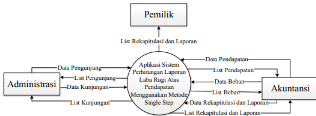
Gambar 1.3 Diagram Konteks Aplikasi Sistem Perhitungan Laporan Laba Menggunakan Metode Single Step
