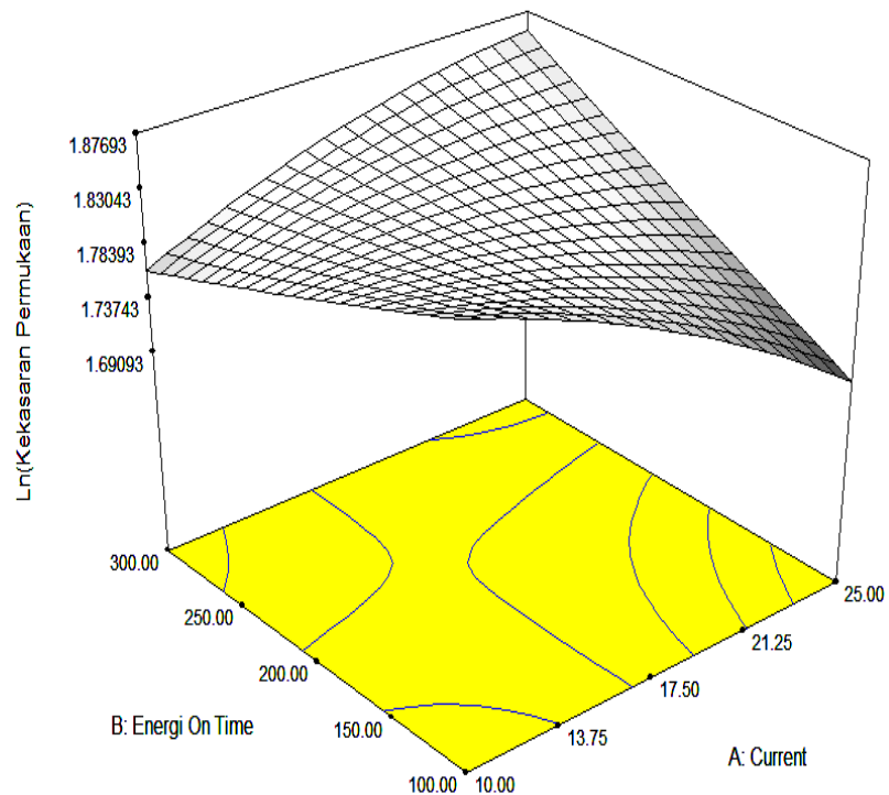
Gambar 11. Plot actual faktor Energy Off Time kekasaran permukaan
