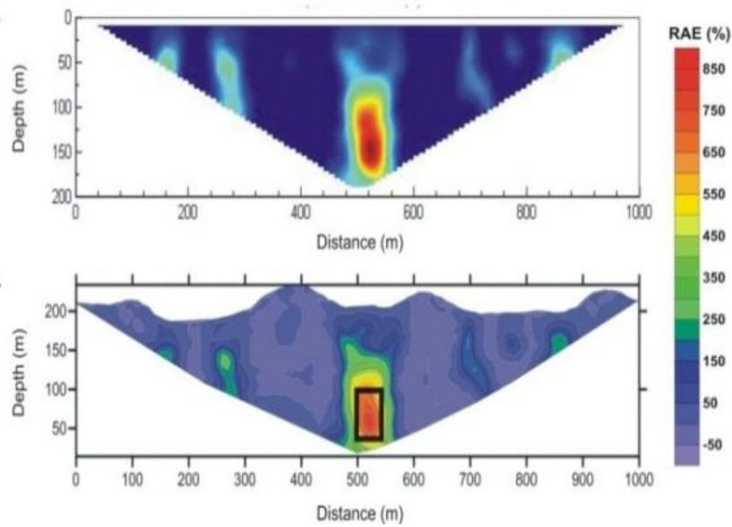
Gambar 8. Hasil pengolahan data VLF lintasan 4, (atas) filter Karous-Hjelt menggunakan matlab, dan (c) Kontur rapat arus terhadap topografi
