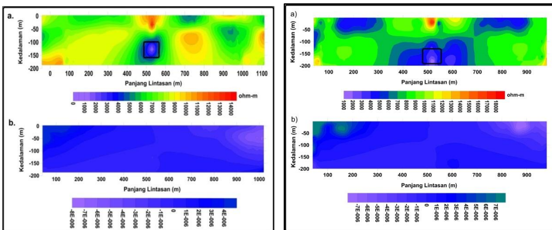
Gambar 12. Hasil pemodelan ke belakang data VLF lintasan 3 (kiri) dan lintasan 4 (kanan) : (a) model resistivitas, dan (b) Model sensitivitas
